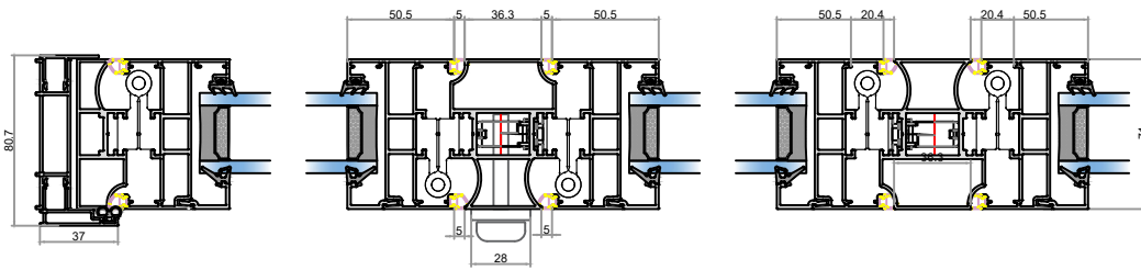
DIŞA AÇILIR
