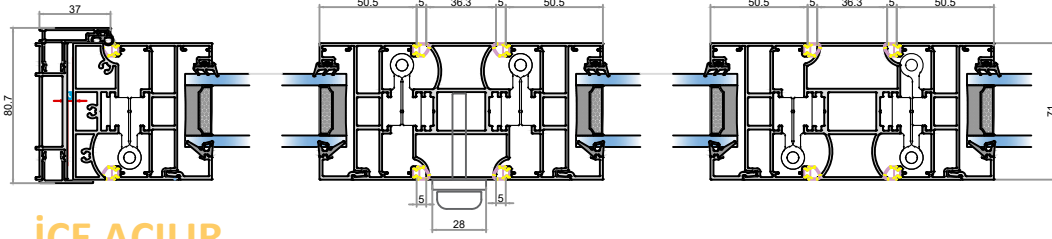
İÇE AÇILIR
